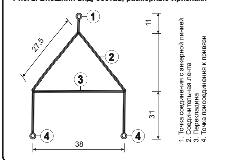
Рис. 3. Совместимое оборудование
